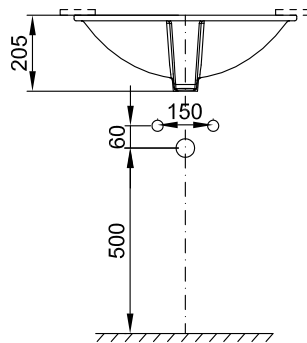
Front view 主视图
