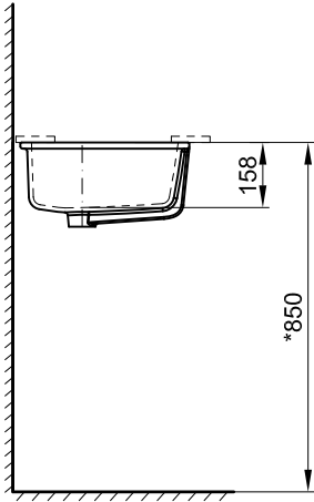
Left view 左视图
