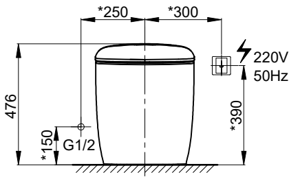
主视图
