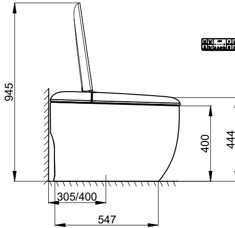
左视图
