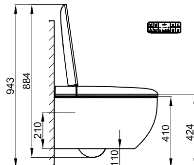
Left view 左视图
