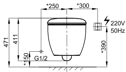
Front view 主视图
