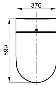
Top view 俯视图
