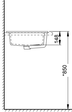
Left view 左视图
