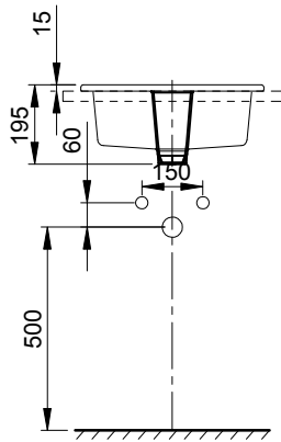
Front view 主视图
