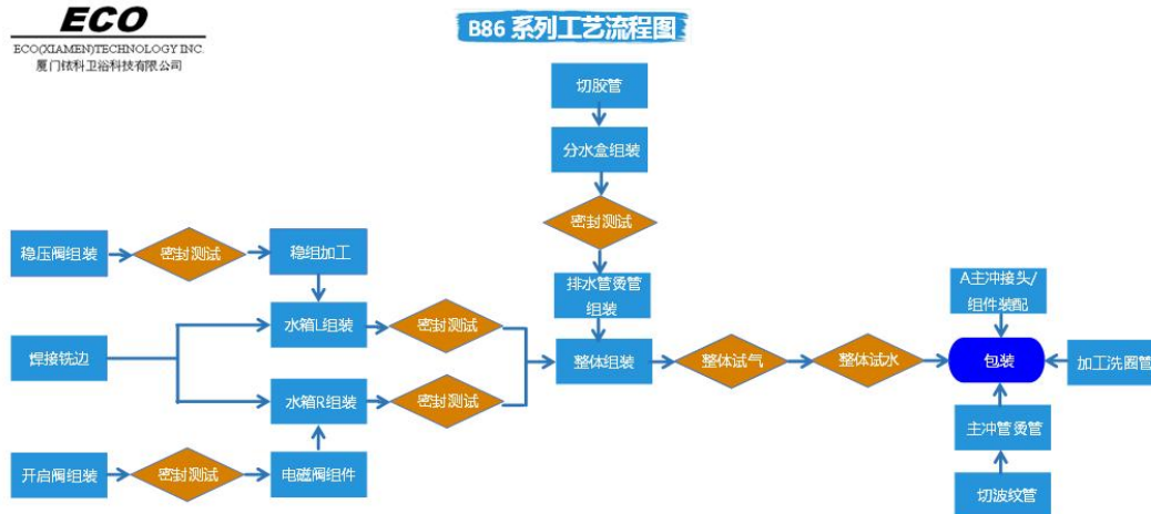
图 3-4 压力包生产工艺流程图
