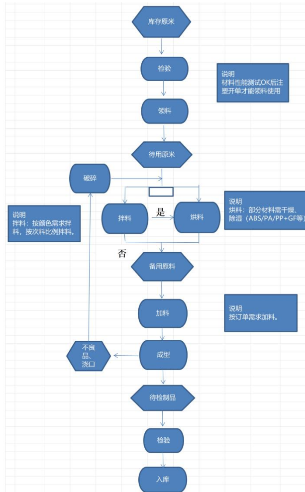
图 3-3 注塑厂生产工艺流程图
