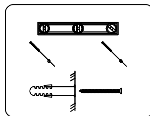
3、固定螺钉 固定好螺钉，螺钉外部预留10-15mm，固定时需要水平尺测量水平
