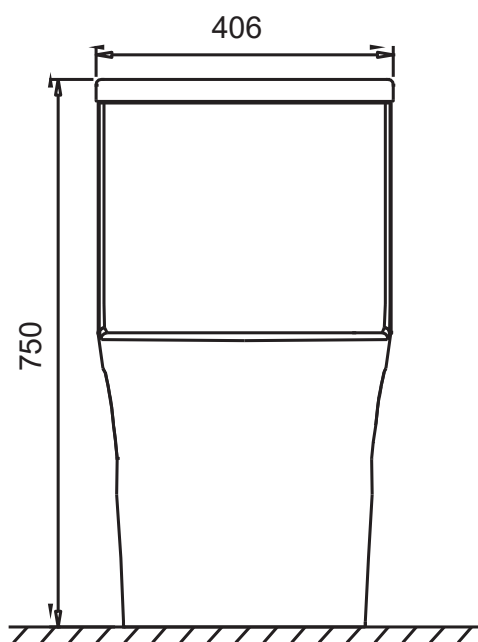
Front view 主视图
