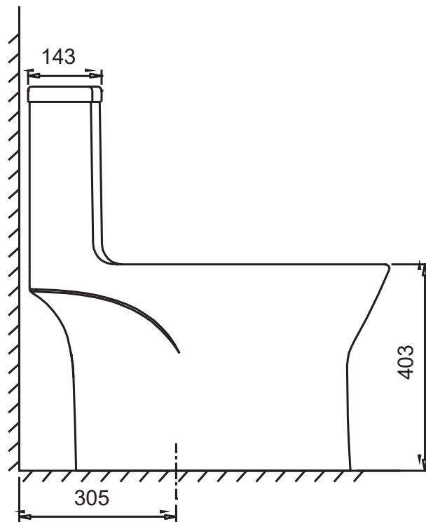
Left view 左视图
