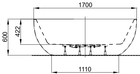
Front view 主视图
