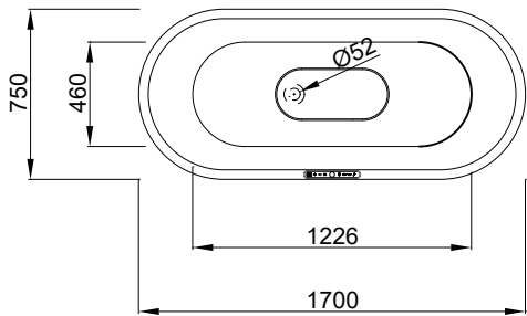
Top view 俯视图
