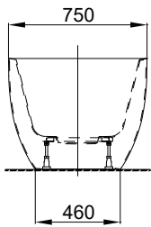
Left view 左视图
