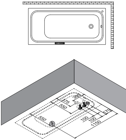
T313-T622右装
