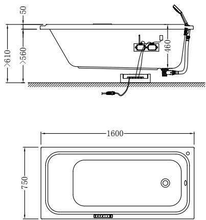
T313-T622右装
