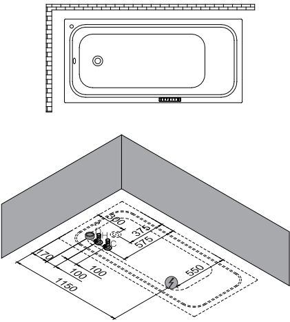
T313-T621左装
