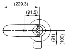
Top view 俯视图
