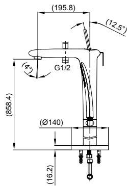
Front view 主视图
