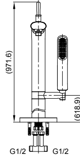
Left view 左视图
