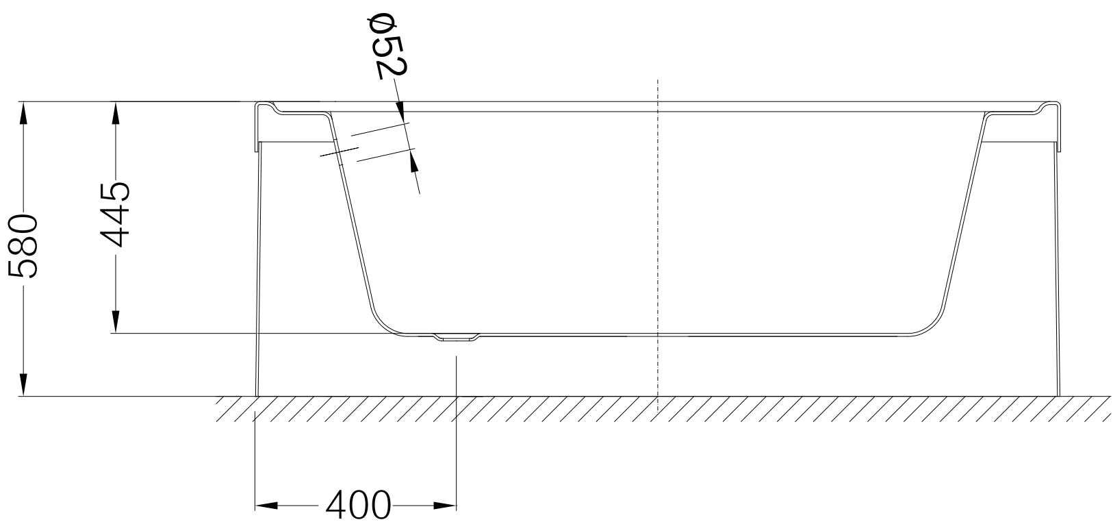
Front view 主视图
