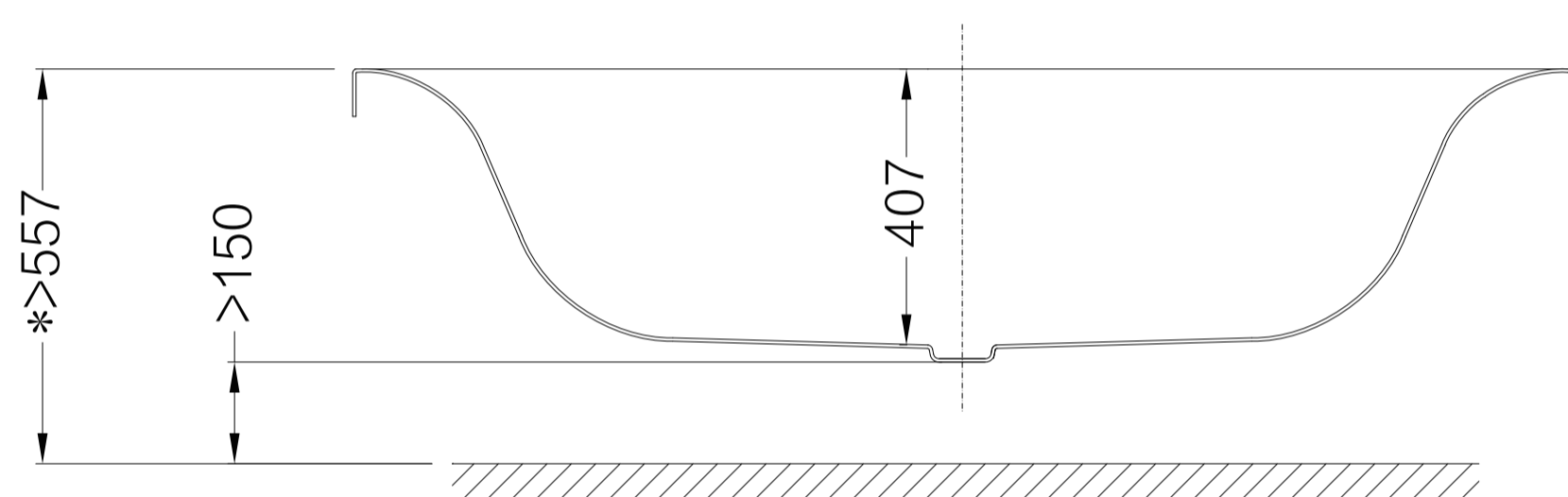
Front view 主视图
