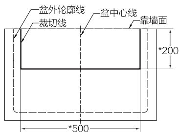
安装尺寸图
