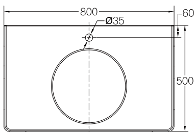
产品尺寸图
